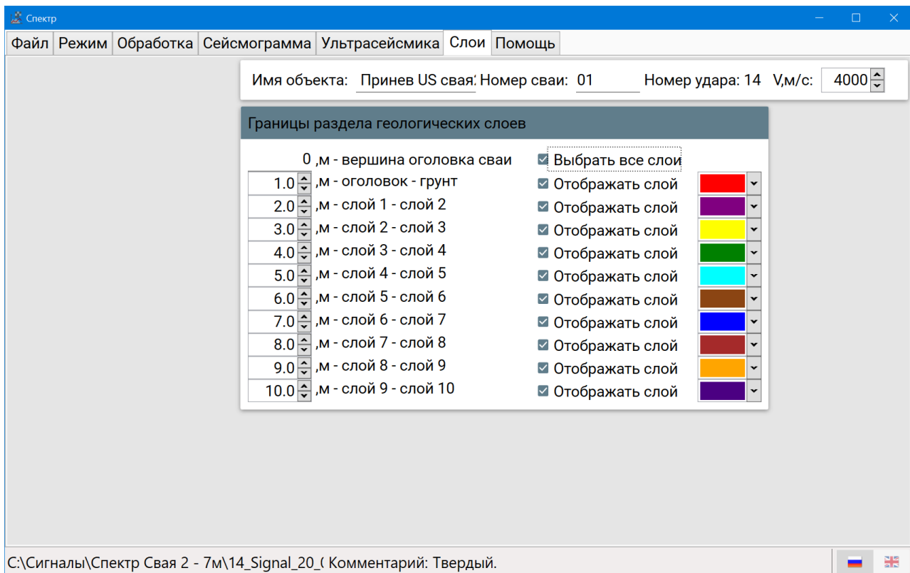
Рисунок А.7 – Работа в меню «Слой»
