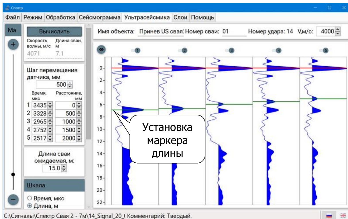
Рисунок А.6 – Работа в меню «Ультрасейсмика»
