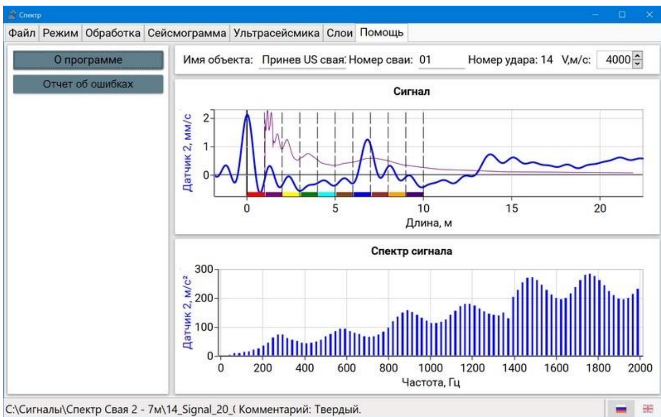
Рисунок А.8 – Работа в меню «Помощь»
