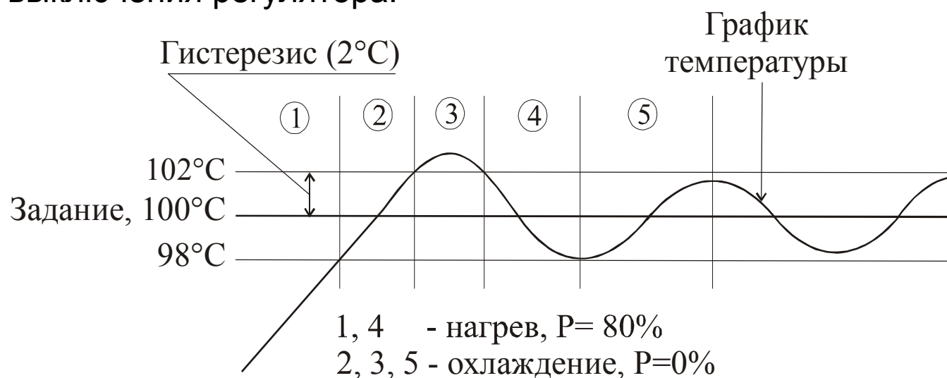
Рис. 4.2. Пример регулирования
