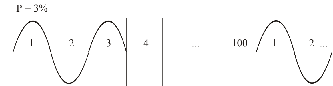
Рис. 4.3. Пояснение работы ШИМ-ограничения мощности
