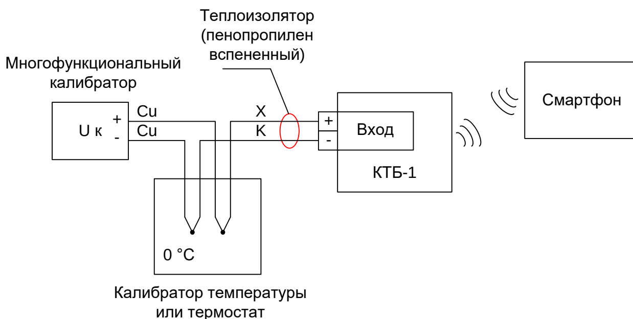
Рисунок 3 – Поверка КТБ-1 с использованием термостата и калибратора напряжений
